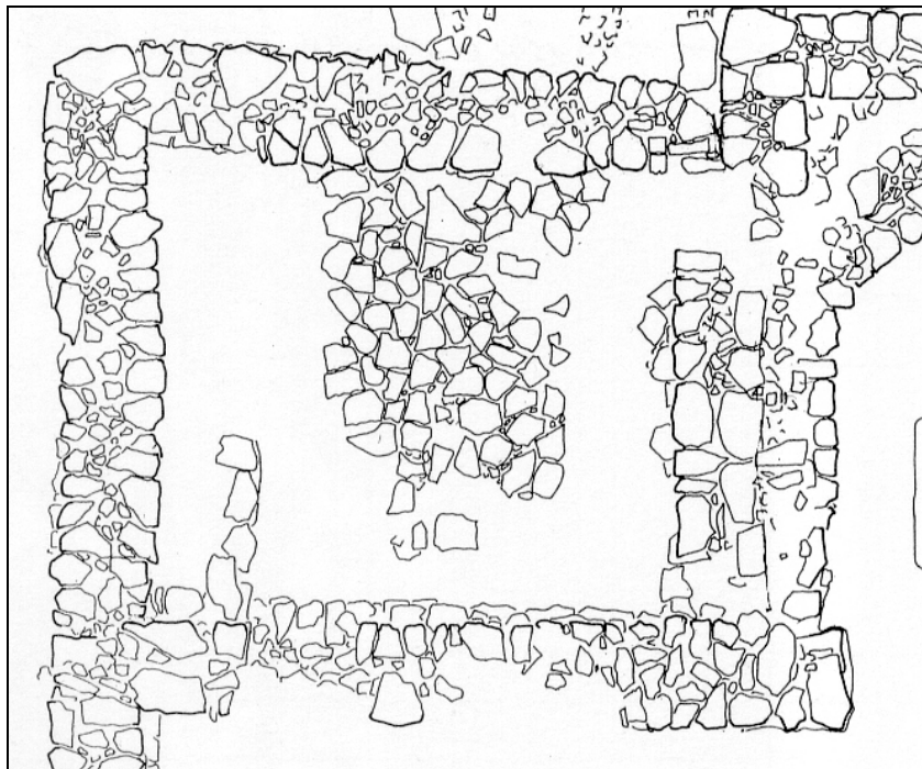
Figura 9. Àmbit Nord de la capçalera de la basílica de Son Peretó (Palol 1994).
